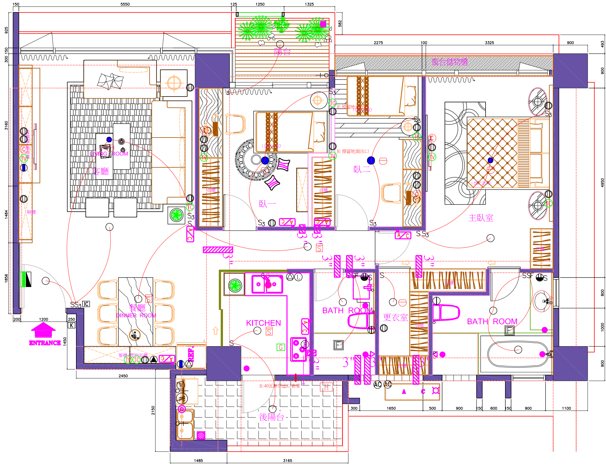
水電圖 SCALE:1/60
